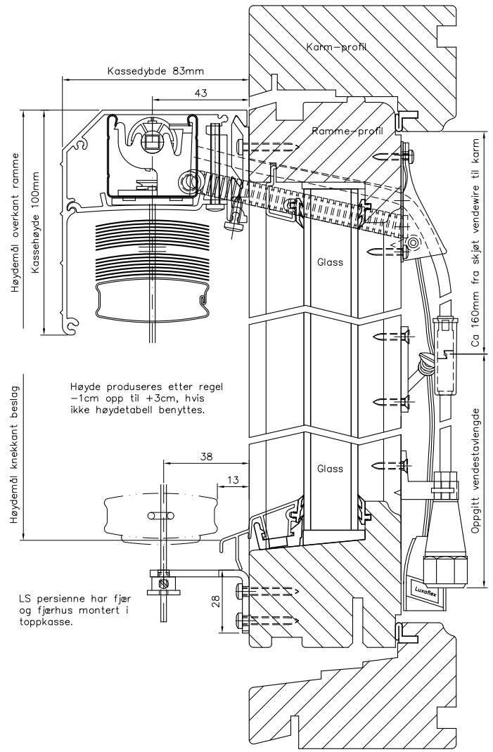
50MM SPESIAL MED EKSTRUDERT KASSE MONTERT PÅ RAMME
